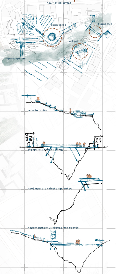
κάτοψη κλίμακα 1:500
