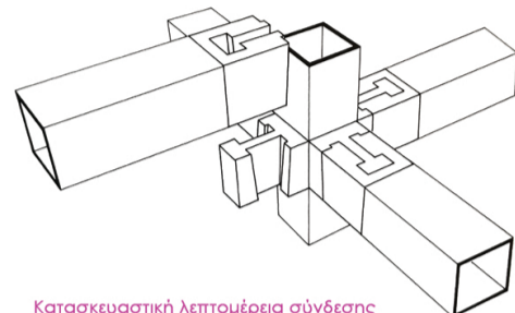
Κατασκευαστική λεπτομέρεια σύνδεσης επέκτασης της μονάδας.
