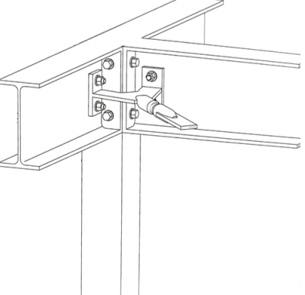
Κατασκευαστική λεπτομέρεια σύνδεσης για την προσθήκη πανέλου προβολών στην έβδομη τυπολογία
