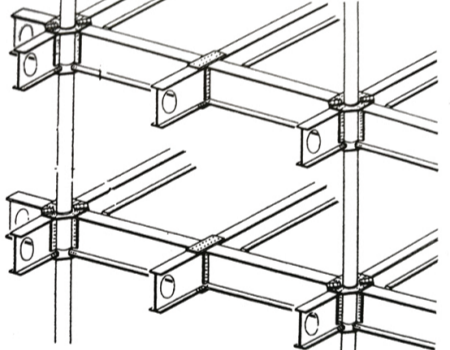
Κατασκευαστική λεπτομέρεια σύνδεσης των καθισμάτων
