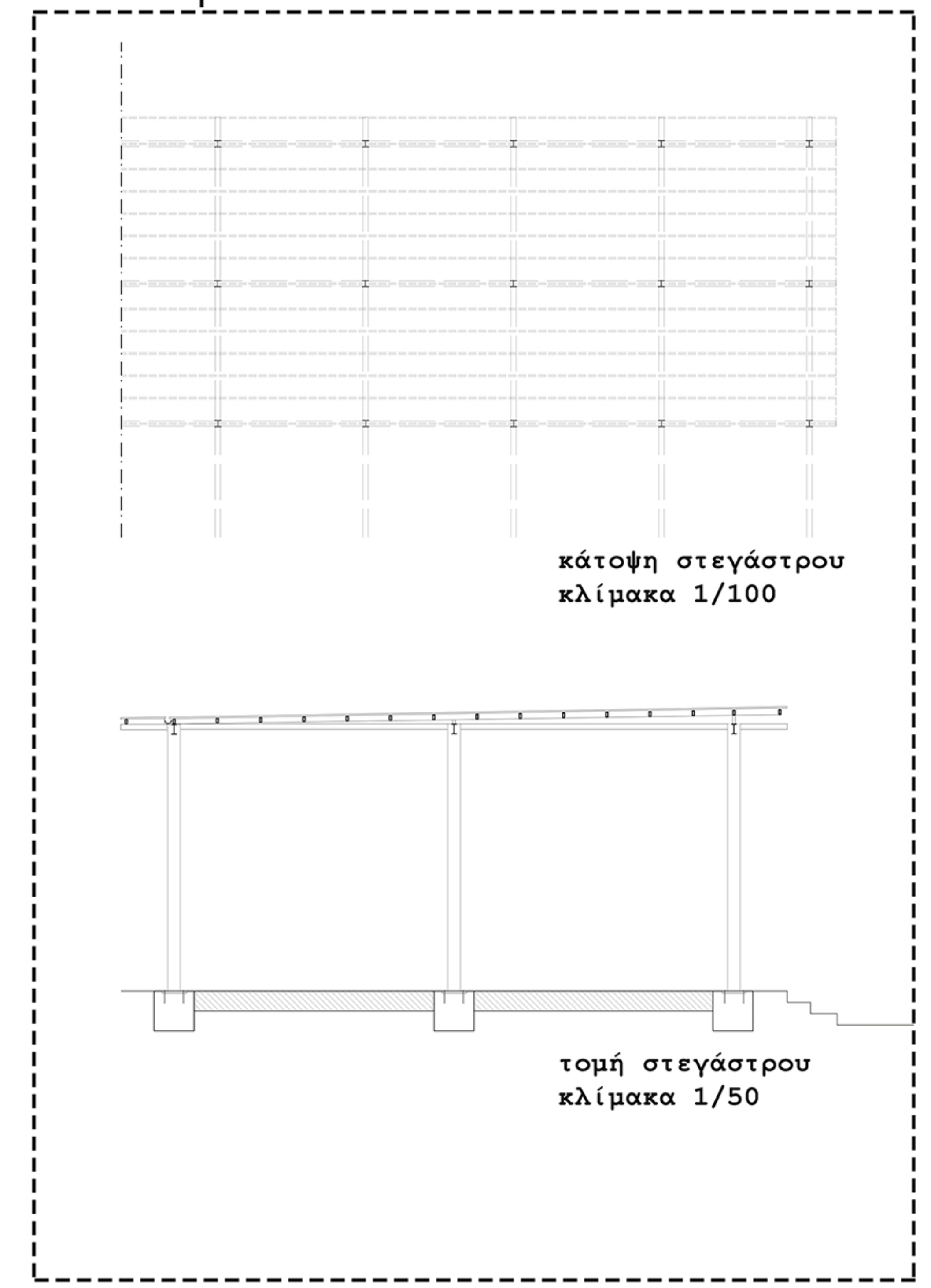
λεπτομέρεια στεγάστρου
